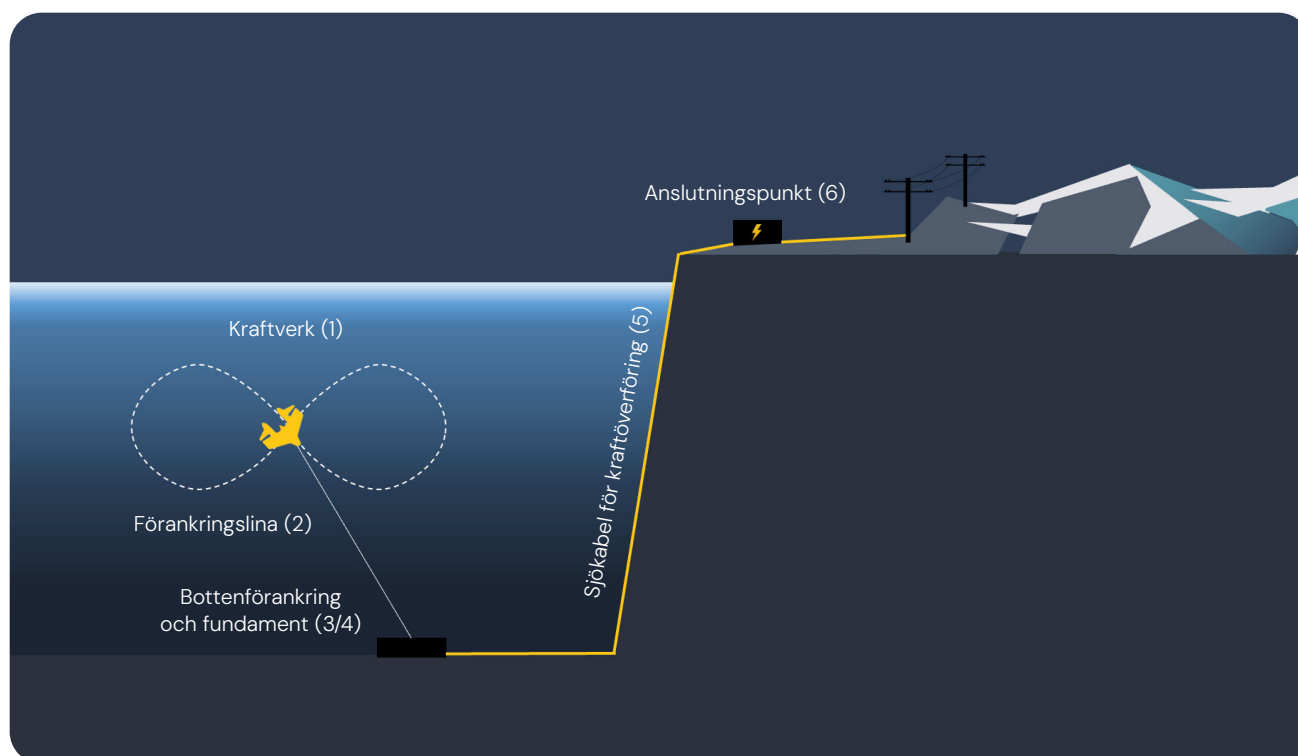
Bild 1. Illustration över de olika delarna vid en installationsplats för Minestos teknik vilka är 1) Kraftverk som genererar elektricitet, 2) Förankringslina som kopplar ihop kraftverket med bottenförankringen, 3) Bottenförankringen som är kraftverkets rotationspunkt, 4) Fundament på havsbotten, 5) Sjökabel för kraftöverföring samt datakommunikation och 6) Anslutningspunkt till elnät. Källa: Minesto
