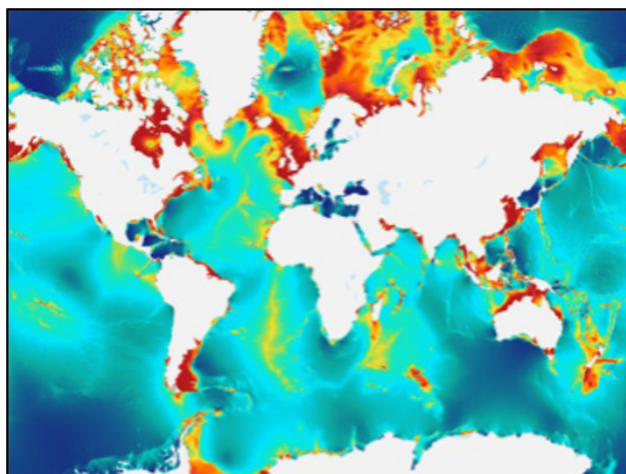
Bild 9 och 10. Karta över oceanströmmar och värmekarta över regioner med höga tidvattenströmmar i världen.
