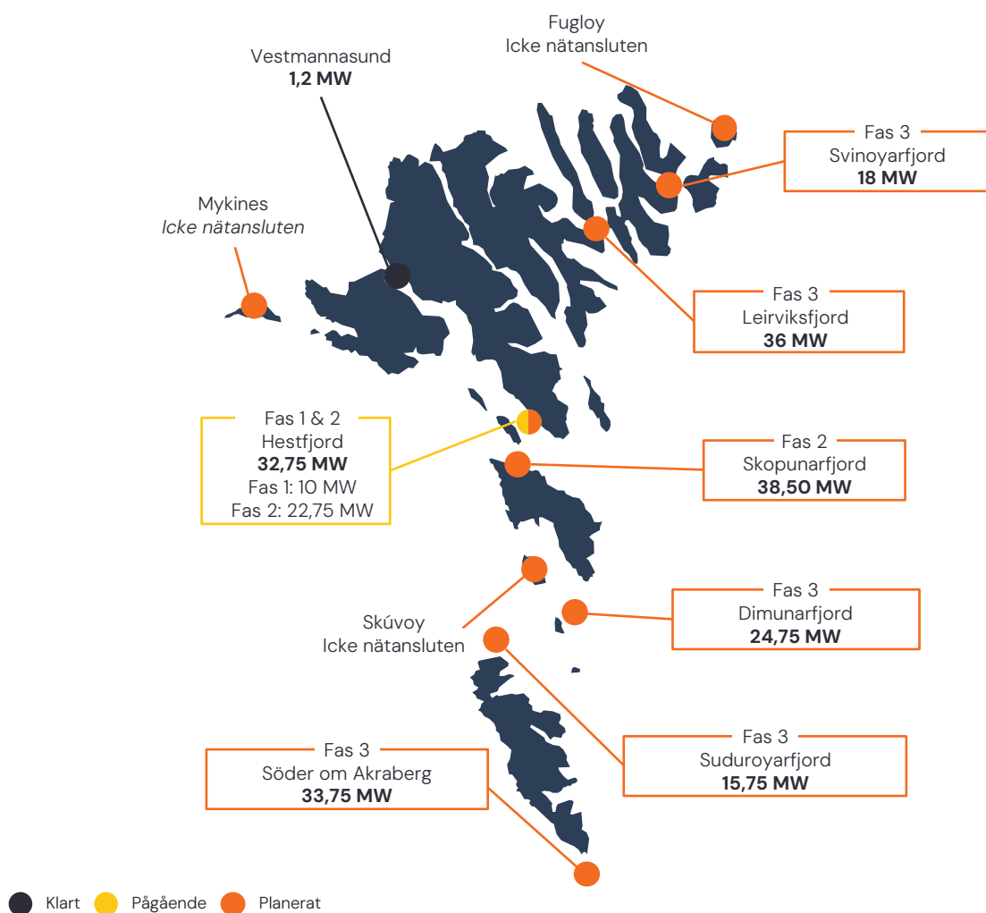
Bild 14. Planerad utbyggnad och faser i Färöarna. Källa: Minesto
