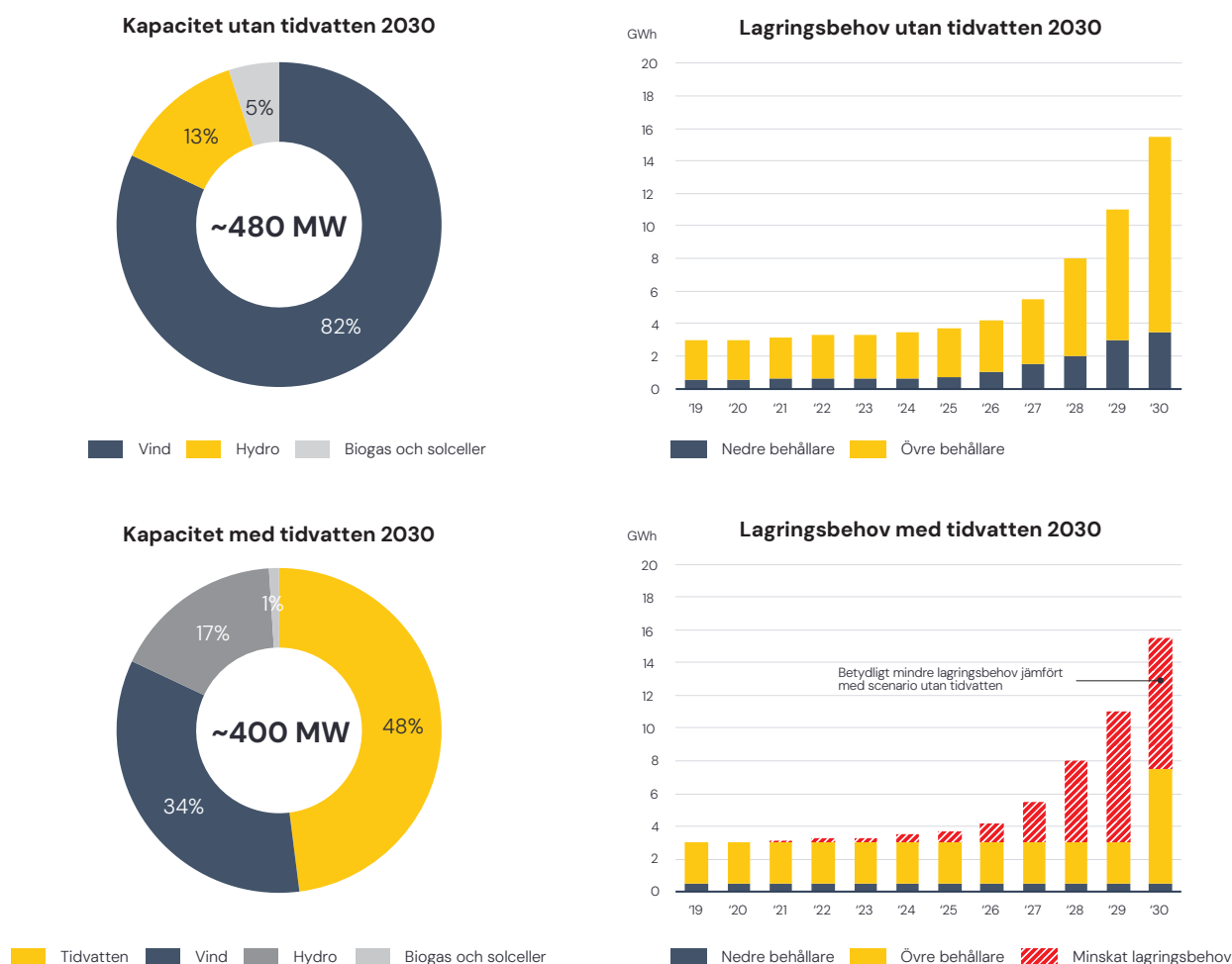
Bild 13. Konsekvenserna för Färöarnas energimix med och utan tidvattenkraft. Källa: Minesto baserat på doktorsavhandling avseende Färöarna. 8
