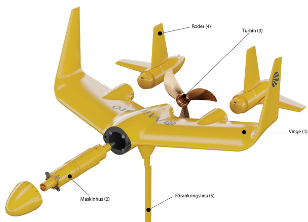
Bild 2. Minestos kraftverk består av 1) en vinge och 2) ett maskinhus innehållande styrsystem och generator. Bakom vingen sitter 3) turbinen och 4) kraftverkets rodersystem. Rodersystemet styr kraftverket automatiskt i en åttaformad bana. 5) En förankringslina kopplar kraftverket till en bottenförankring i ett fundament på havsbotten. Förankringslinan rymmer elkablar såväl som kablar för kommunikation. Källa: Minesto
